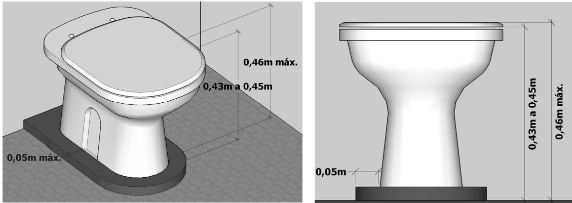
Figura 2. Adequação de altura da bacia sanitária com sóculo
