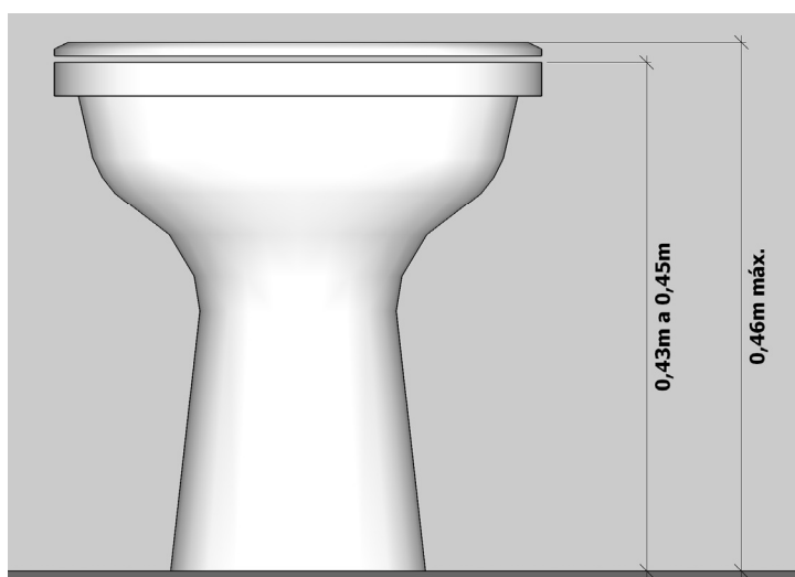
Figura 1. Vista frontal da bacia sanitária
