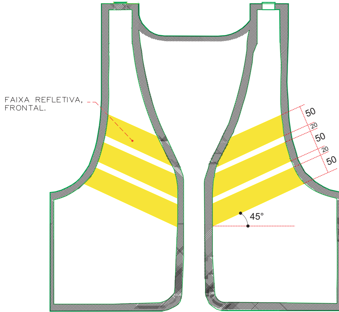
VISTA FRONTAL. Sem escala
