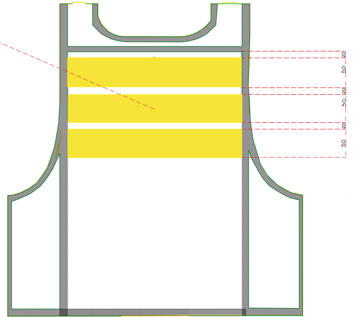
VISTA TRASEIRA. Sem escala
